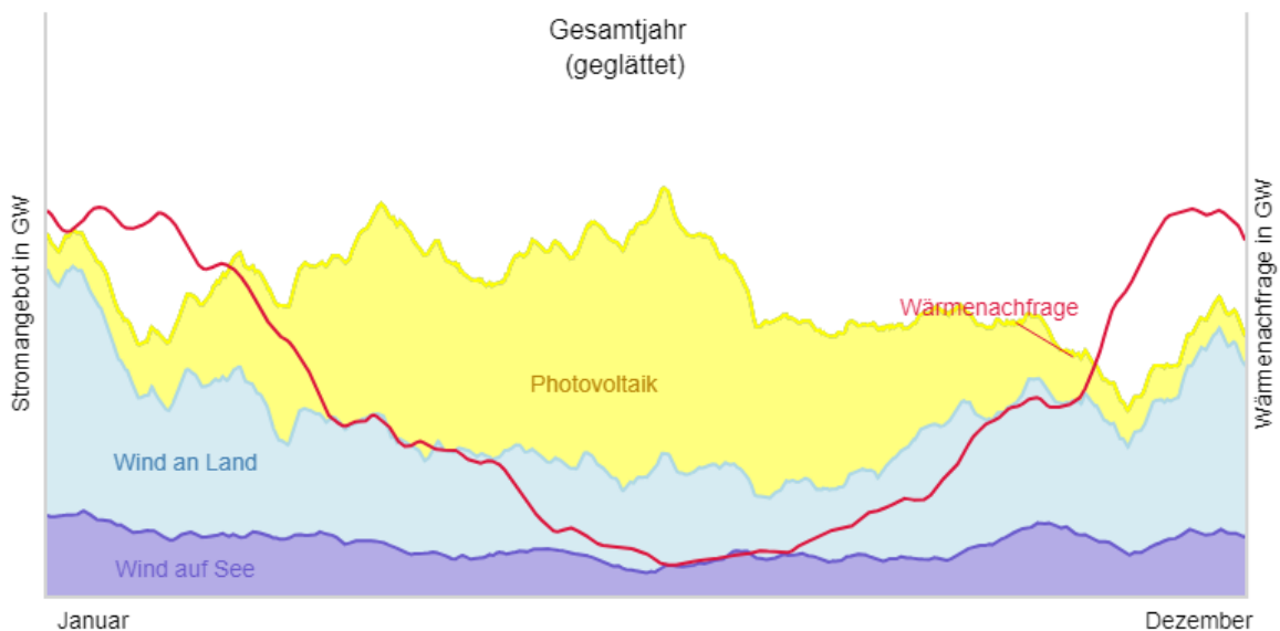
Abbildung 1: Schematische Darstellung des Angebots an EE-Strom (linke Achse), sowie der Wärmenachfrage (rechte Achse) im Jahresverlauf. Quelle: Eigene Darstellung.
