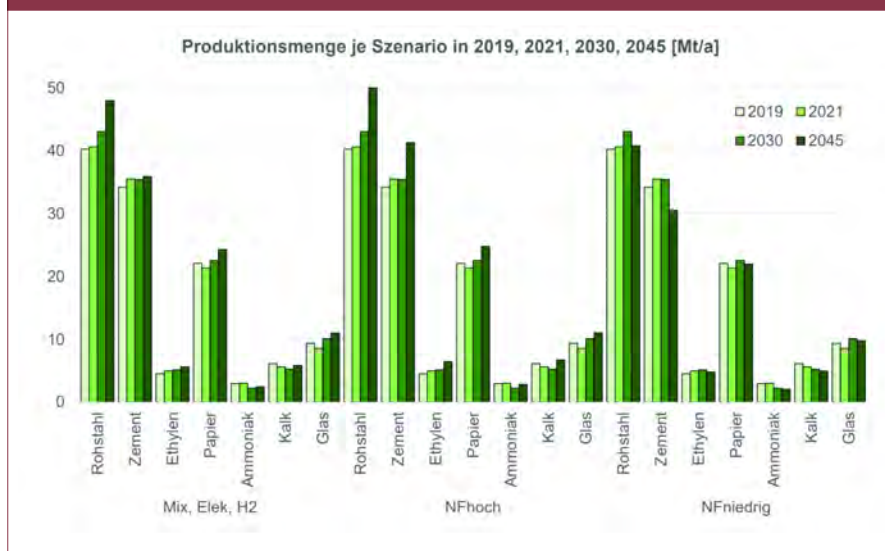
Abbildung 5.2: Produktionsmenge in Mt je Szenario für die Jahre 2019, 2021, 2030 und 2045.
