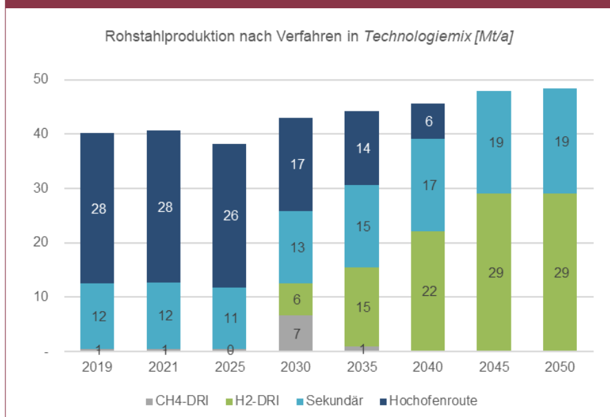
Abbildung 5.3: Rohstahlproduktion nach Verfahren im Mix-Szenario.
