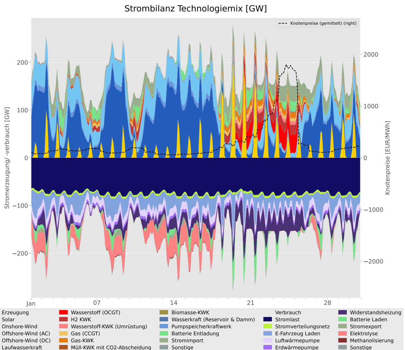
Abbildung 6.5: Stromerzeugung und -verbrauch in Drei-Stunden-Schritten im Beispielmonat Januar (Wetterdaten von 2019) im Szenario Technologiemix im Jahr 2045 für das Modell PyPSA-DE.
